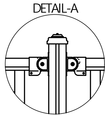
연결상세도
